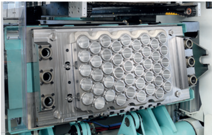
Stampo a 45 cavità. 45-cavities mould.
